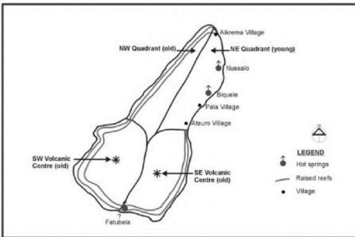
Figura 20 Mapa de fonte hidrotermal da ilha de Ataúro. (Lawless et al, 2005):
