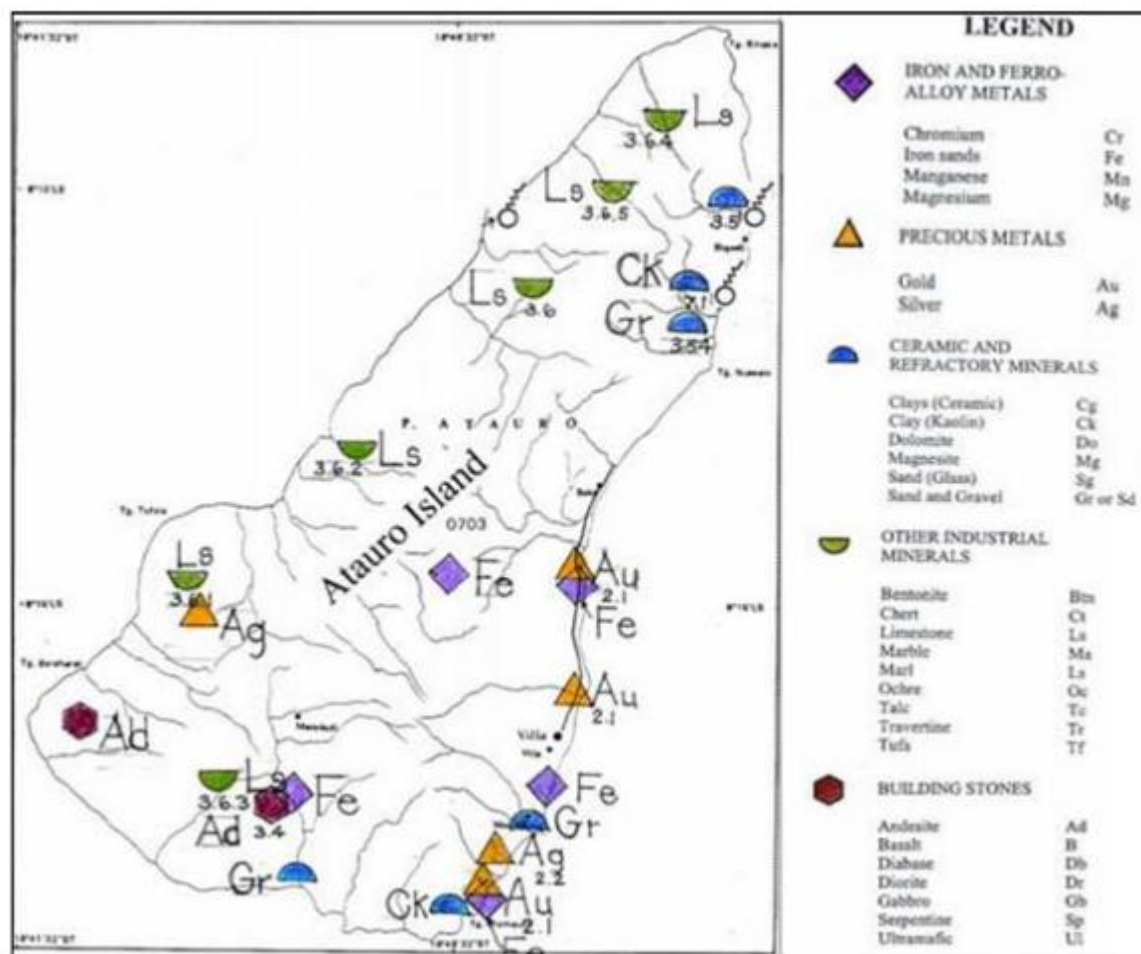
Figura 22 Mapa de distribuição dos recursos minerais da ilha de Atauro. (Fonte: Adotado de Jhon L. Rau, 2002)
