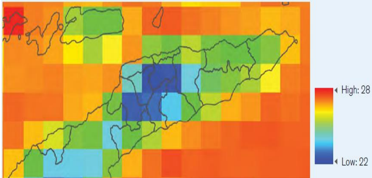
Figura 18 Informasaun temperatura anuál, bazeia ba data istóricu temperatura °C husi 1991-2022 ba Timor-Leste (ERA5-dataset), (Fonte: World Bank, 2025).
